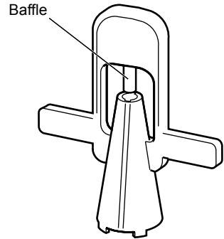
Vaporiser head
